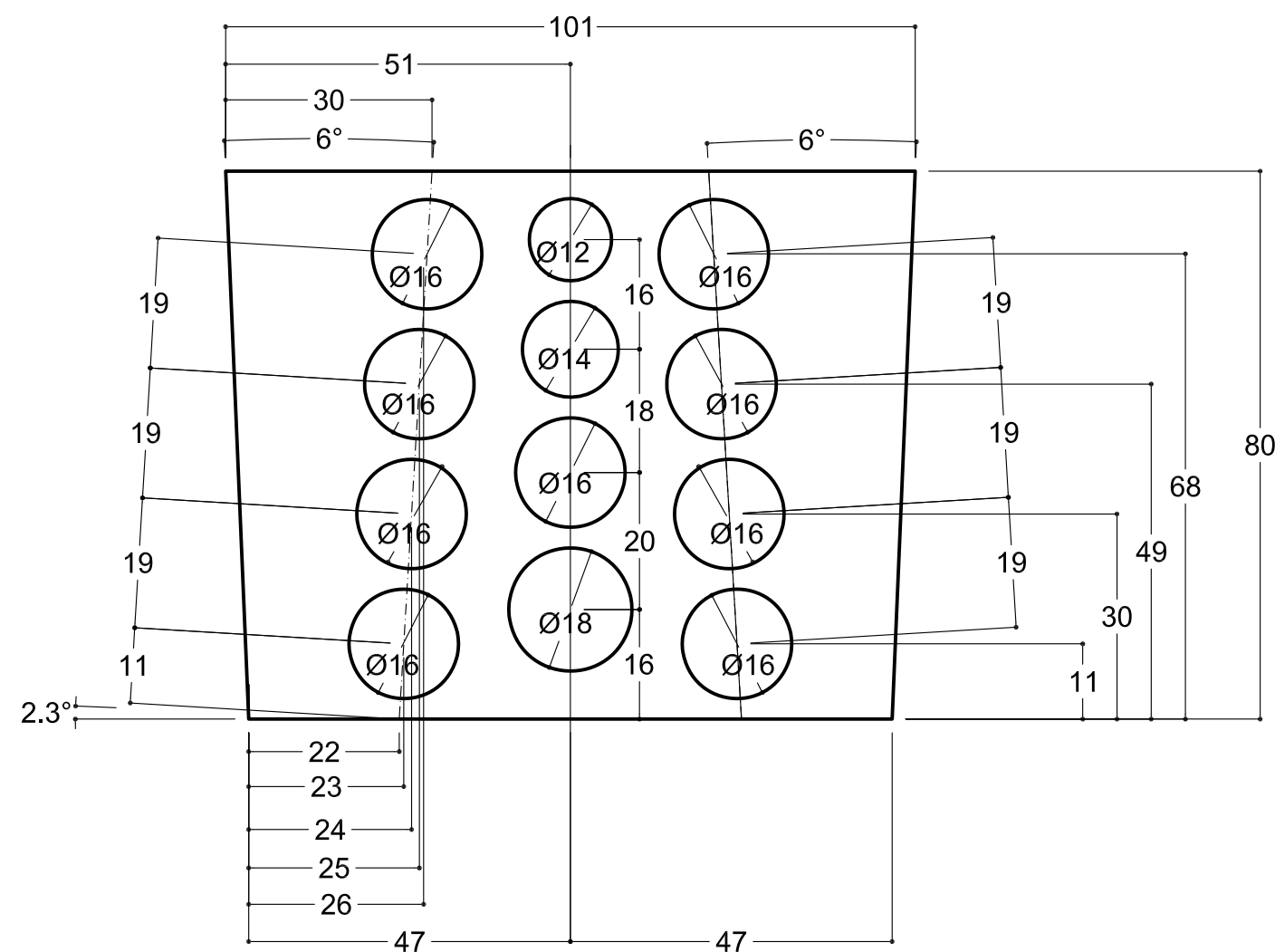
VISTA FONDO
